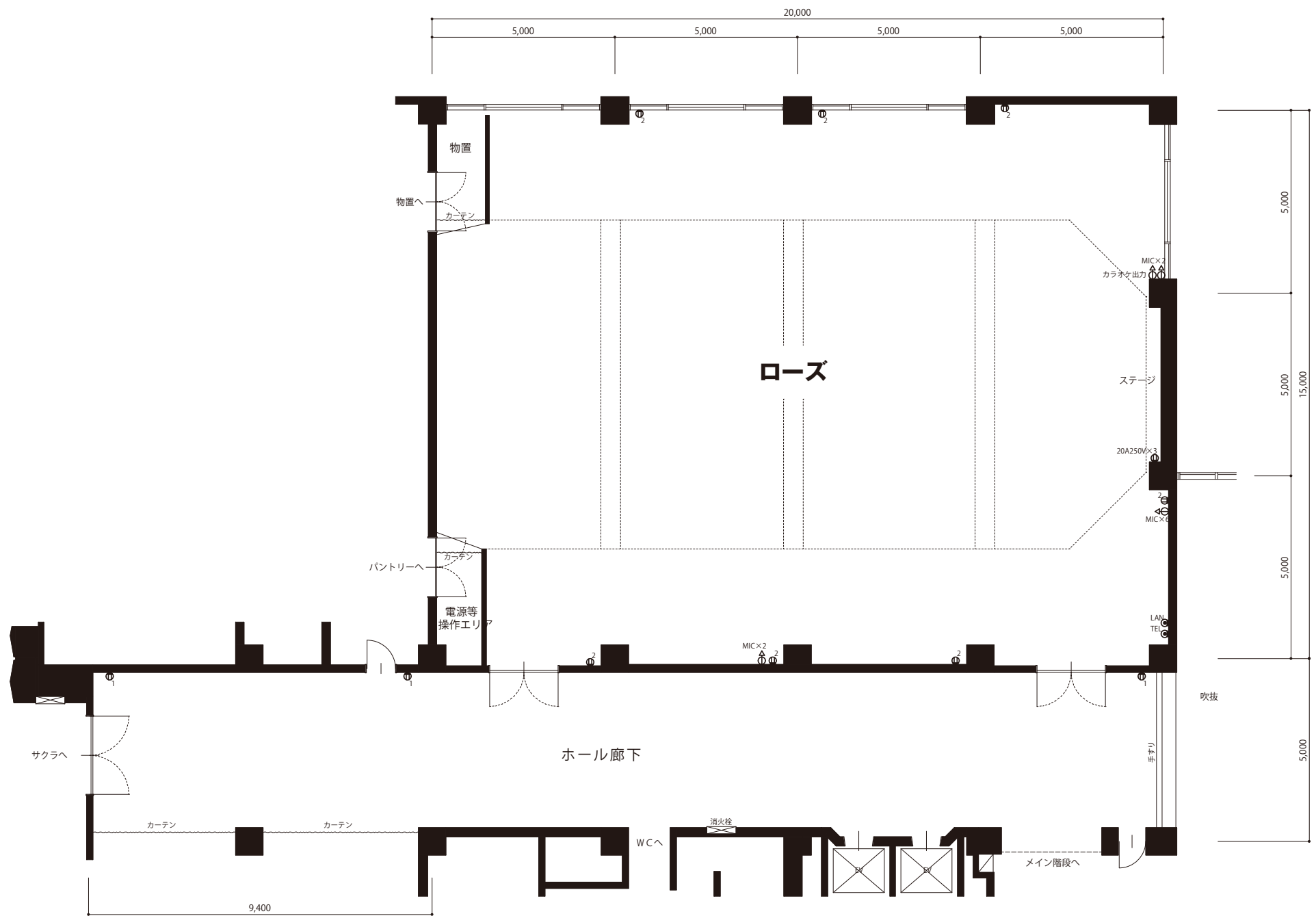
ローズ 詳細図
